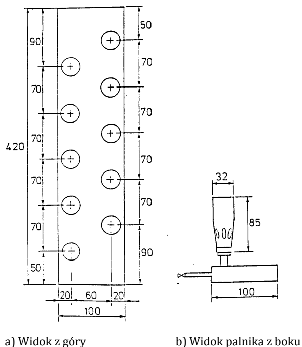
Rys. 1. Zespół palników
