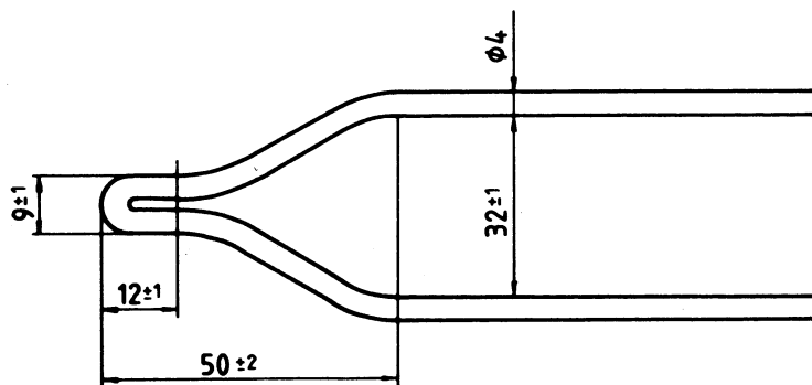
Rys. 2.25.3-1. Pętla żarowa (wymiarów w mm)
