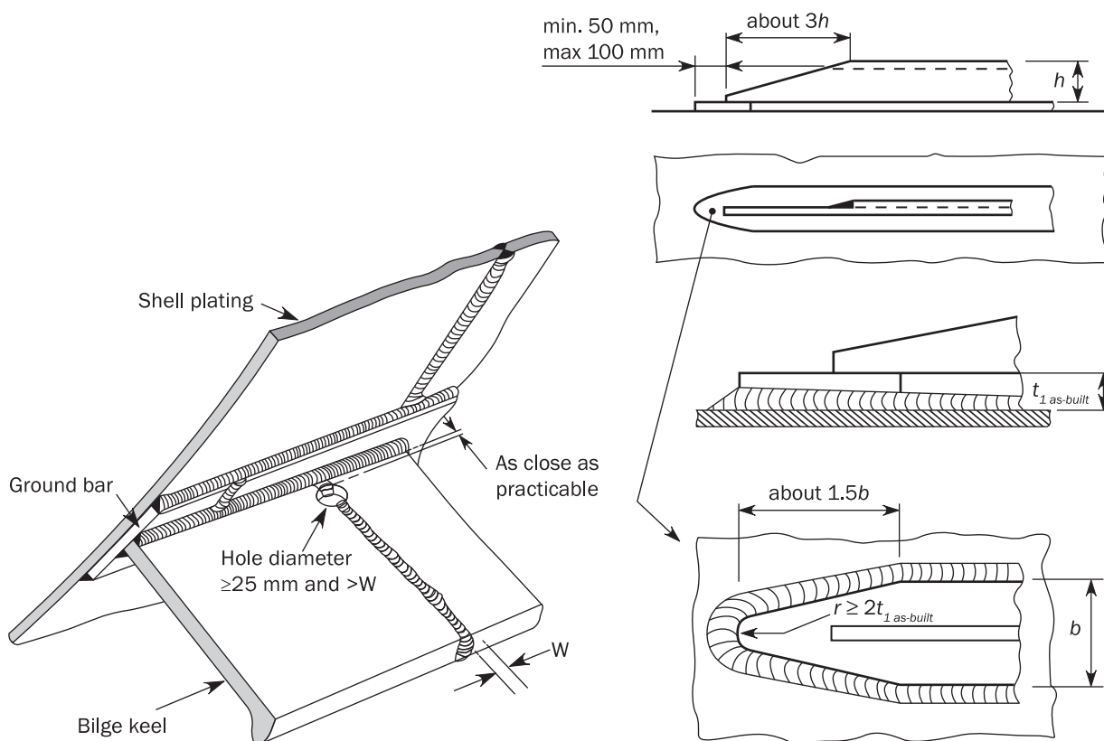
Figure 10 : Bilge keel
