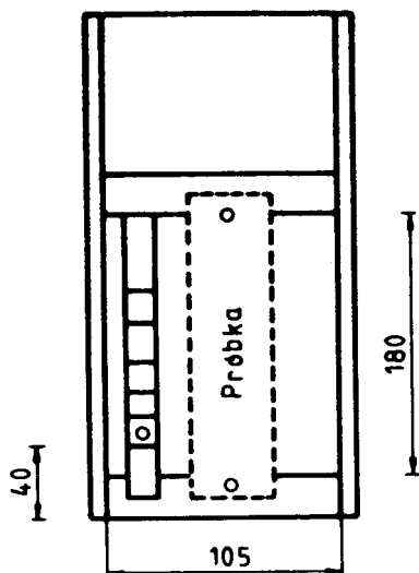
Rys. 2.20.3-3 Uchwyt próbki ze skalą (wymiary w mm)
