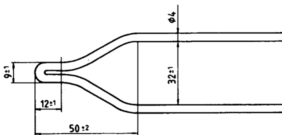
Rys. 2.20.3-1 Pętla żarowa (wymiary w mm)
