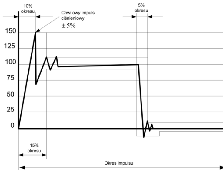
Rys. 2.3.1 Przebieg impulsu ciśnieniowego
