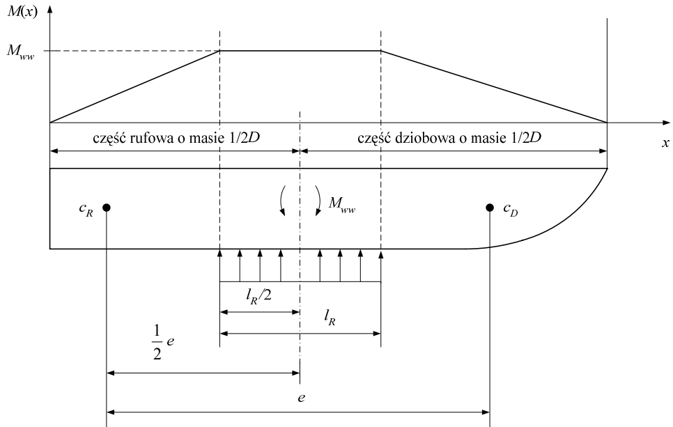
Rys. 6.5.2.2 Zginanie ogólne powodujące wygięcie kadłuba
