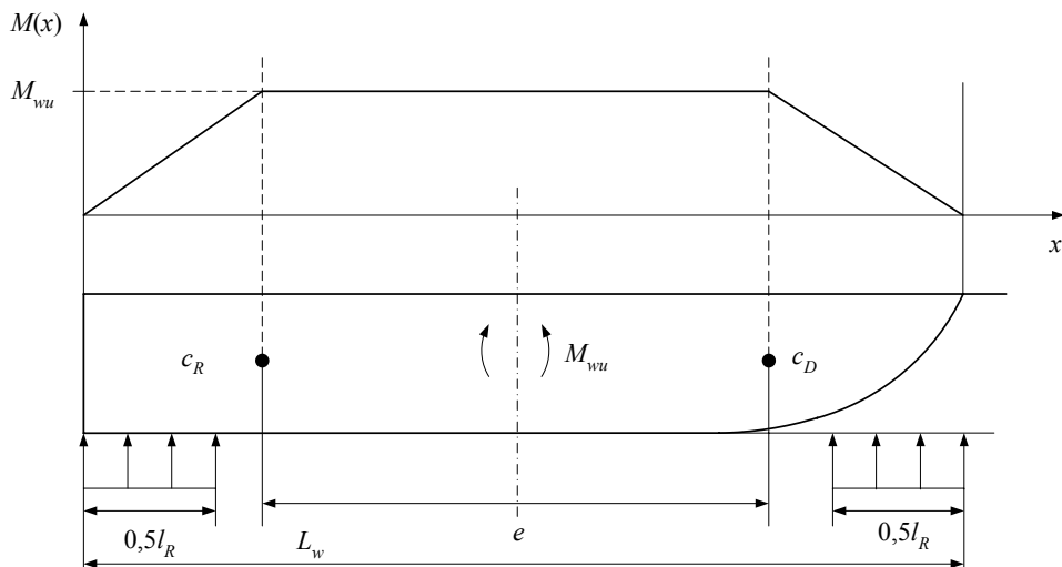
Rys. 6.5.2.3 Zginanie ogólne powodujące ugięcie kadłuba
