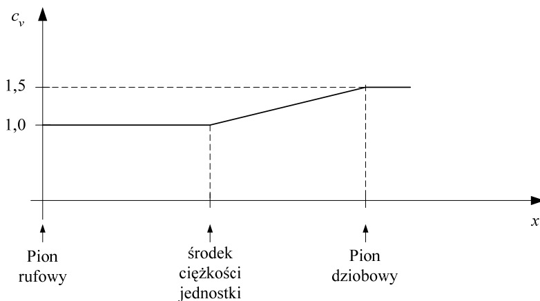
Rys. 5.2.1.4 Wartość c_v
