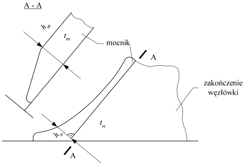
Rys. 7.2.2.4 Zakończenie węzłówki
