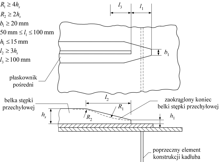
Rys. 7.3.1.2 Zalecana konstrukcja stępki przechyłowej
