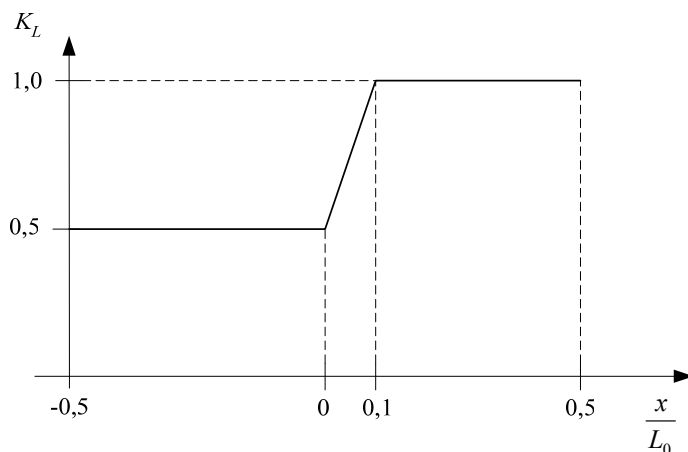
Rys. 5.3.2.2 Wartość współczynnika K_L
